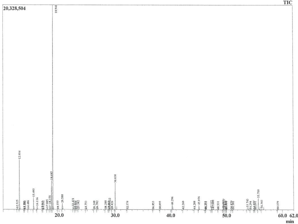
Chromatogram Melaleuca quinquenervia
